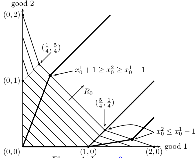
Figure 4: Lemma 9.
